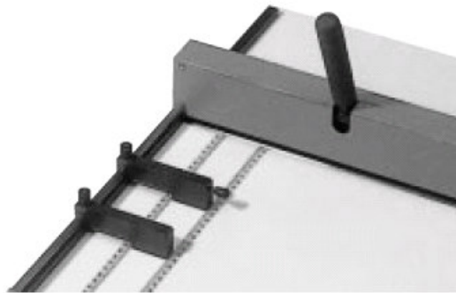
RILLNAK 52 Afmetingen / Dimensions : H/H 120 x B/L 555 x D/P 750 mm
